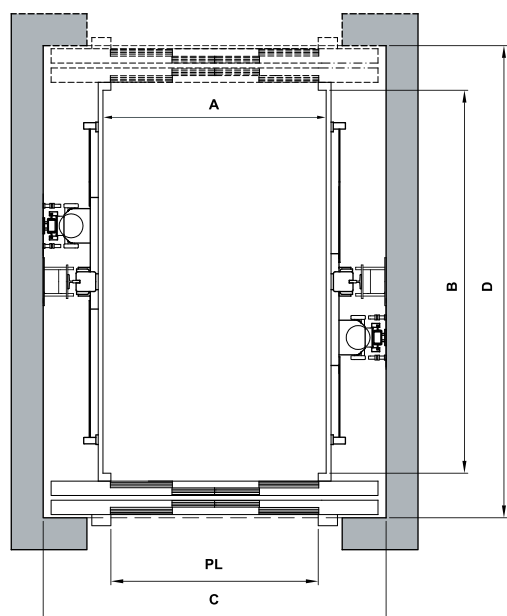
PIANTA VANO
