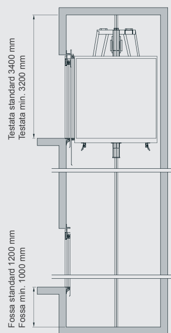
SEZIONE VERTICALE
